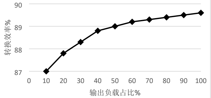
负载效率曲线
