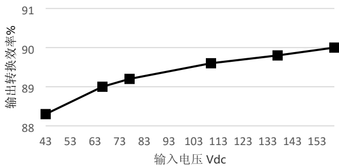
输入电压效率曲线
